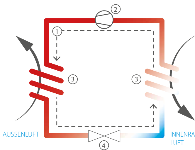
KÜHLZYKLUS
