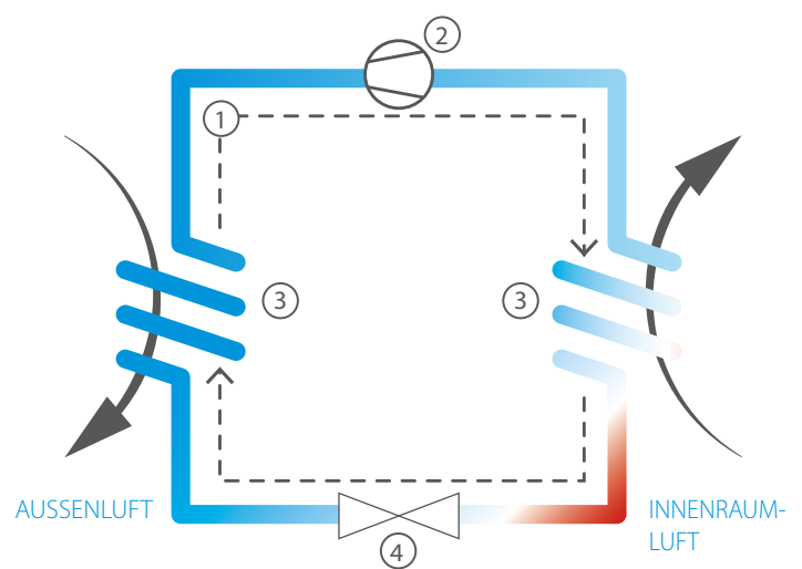
HEIZZYKLUS
