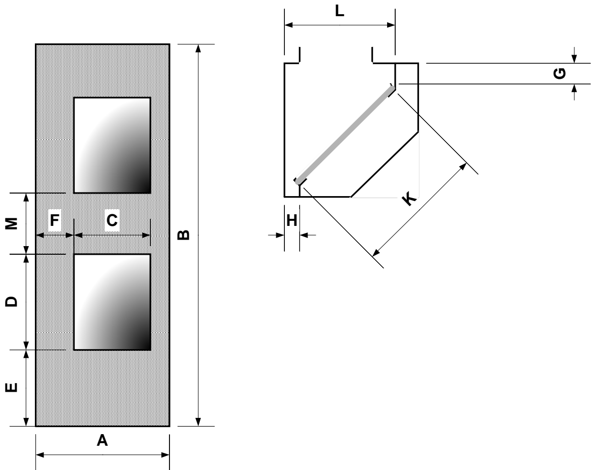
Haubenabmessungen
