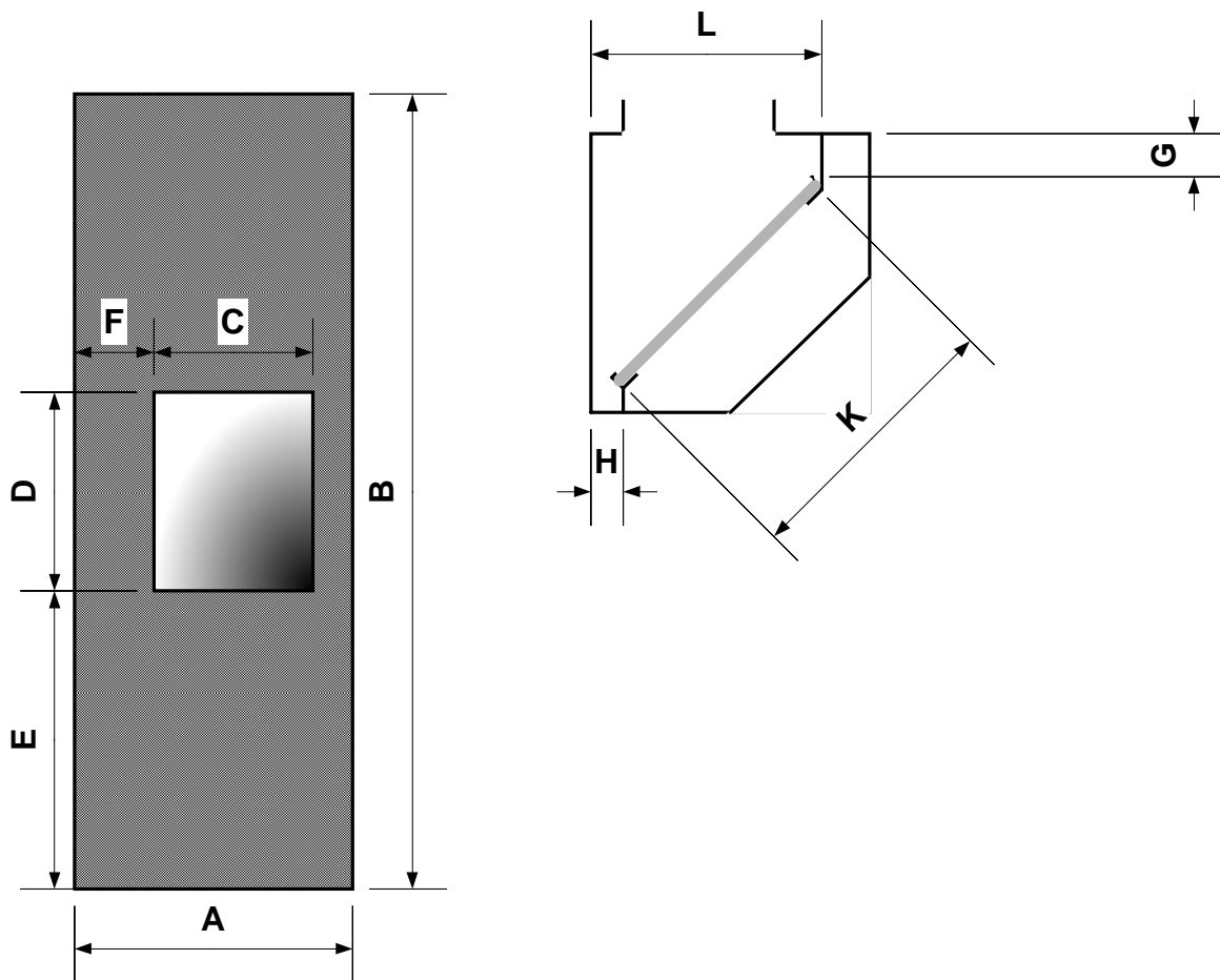
Haubenabmessungen
