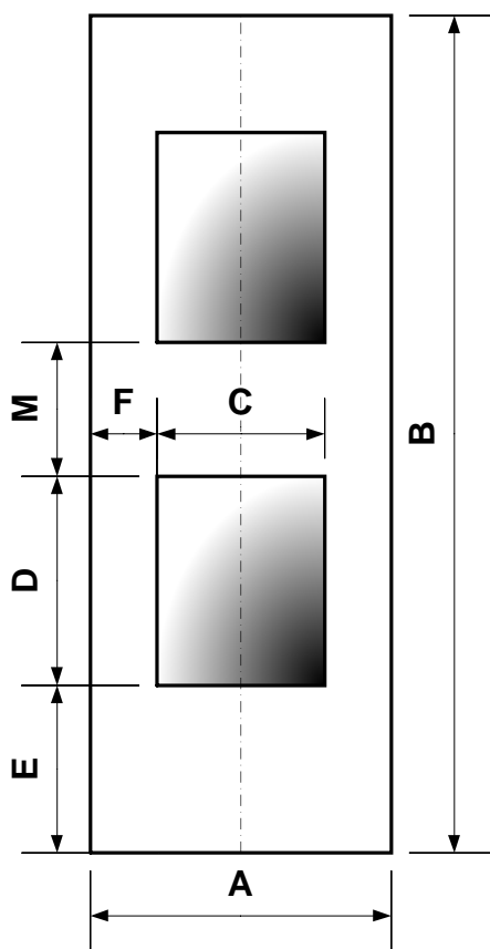
Haubenabmessungen
